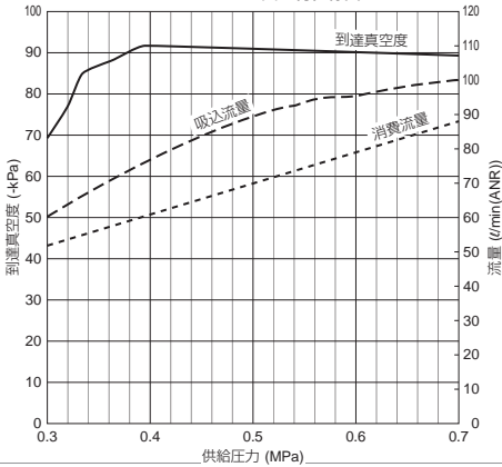
VQD12□-□□□□-□-□真空特性線図
