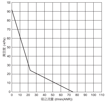
VQD12□-□□□□-□-□流量特性線図
