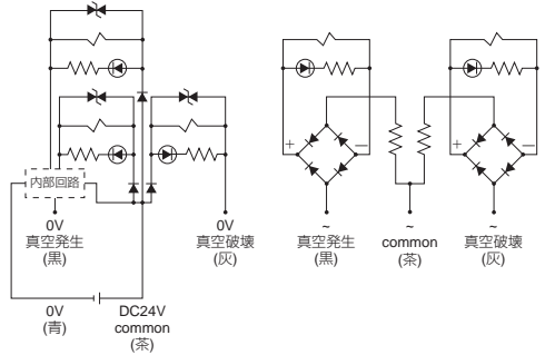
ツインノズルタイプ
