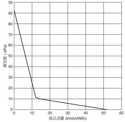
VQD10□-□□□□-□-□流量特性線図
