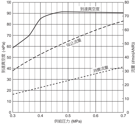
VQD10□-□□□□-□-□真空特性線図
